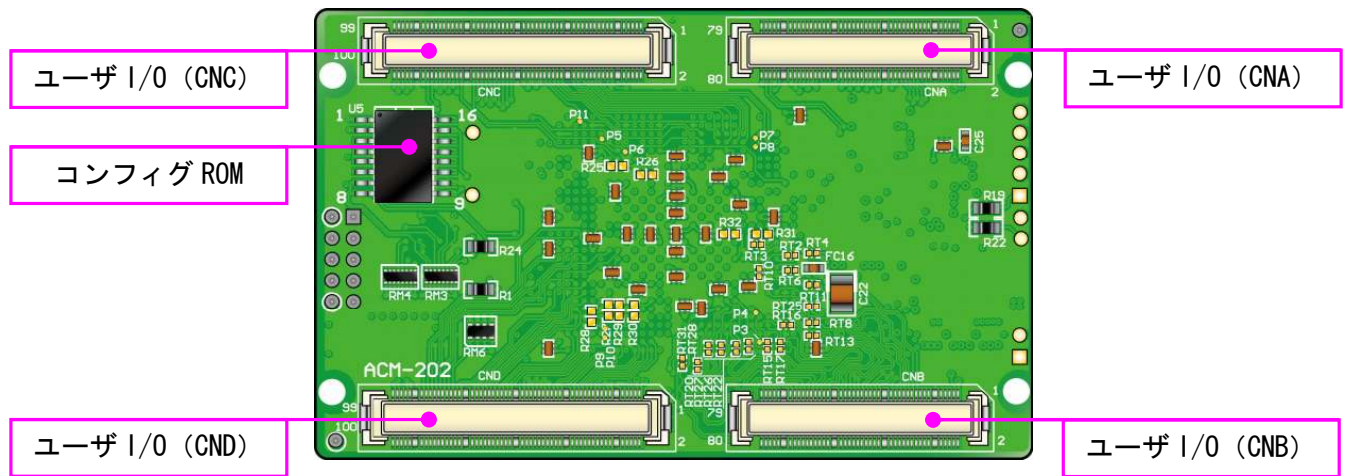
はんだ面
