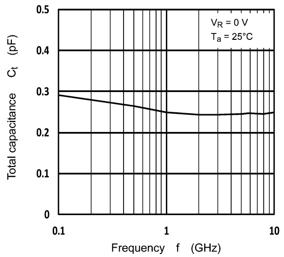
図 8.4 C_t - f
