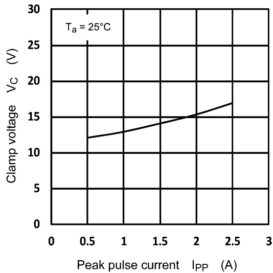
図 9.1 V_C - I_{PP}
