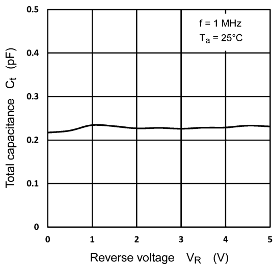
図 8.3 C_t - V_R
