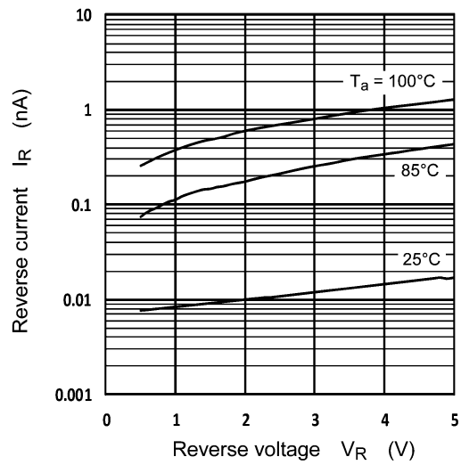
図 8.2 I_R - V_R
