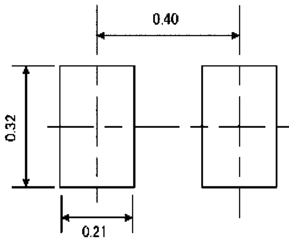
図 7.1 参考パッド寸法 (Unit: mm)
