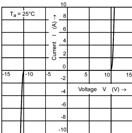
図 8.1 I - V
