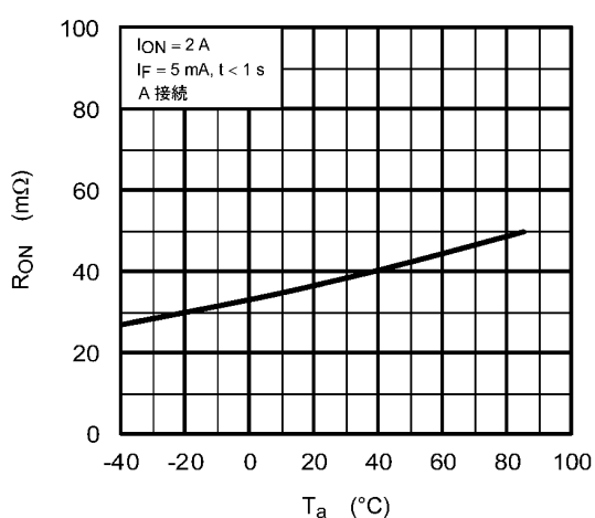
図 12.1.5 R_{ON} - T_a
