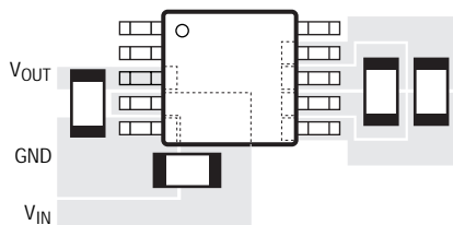
図6．推奨レイアウト
