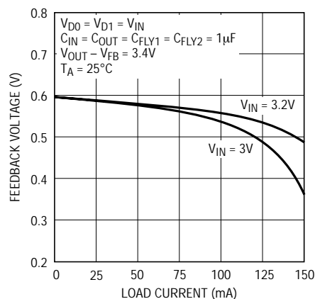
V_{FB} と負荷電流
