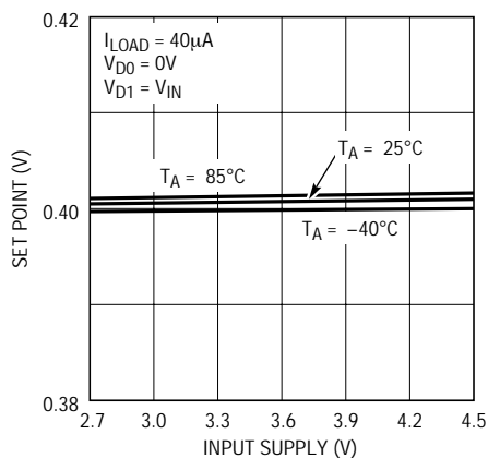
V_{FB} セットポイントと入力電源 (400mV設定)
