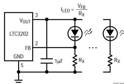
図1. 電流制御モード
