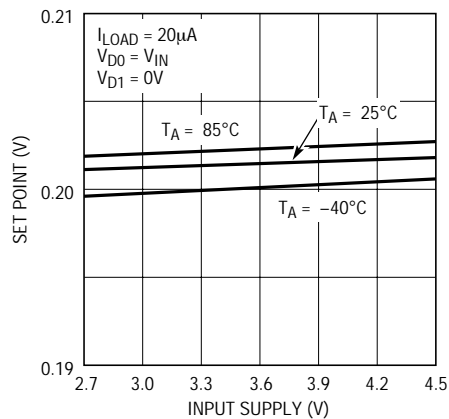
V_{FB} セットポイントと入力電源 (200mV設定)
