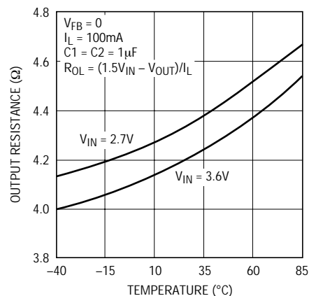
図4．標準的 R_{OL} と温度
