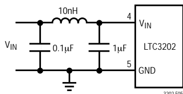
図5 . 10nHのインダクタを使った入力ノイズの低減
