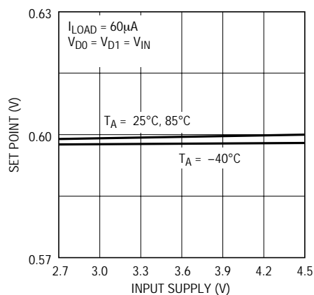
V_{FB} セットポイントと入力電源 (600mV設定)
