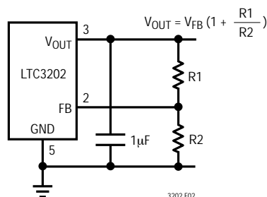
図2．電圧制御モード
