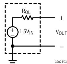
図3．等価開ループ回路
