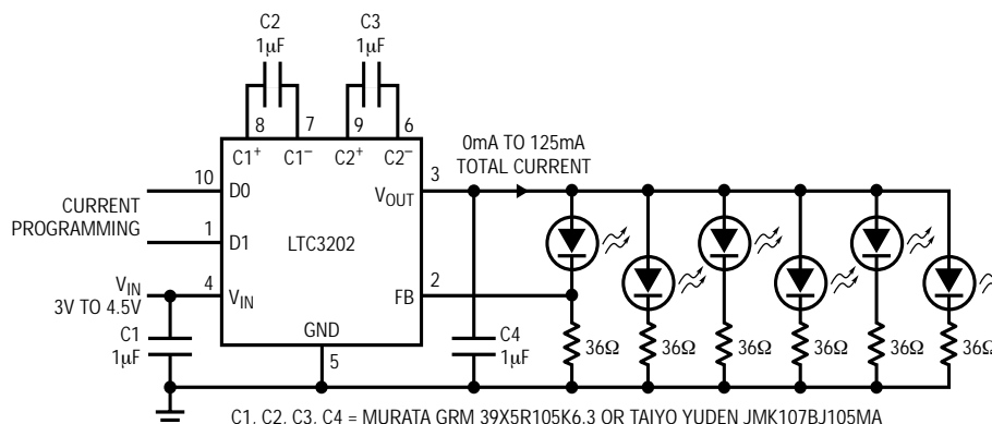
プログラミング可能な白色LED電源
