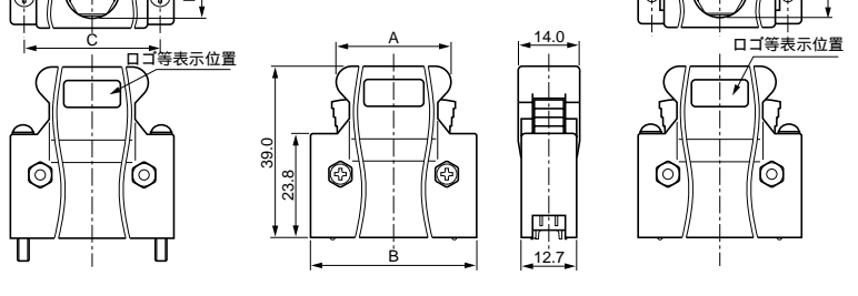
ワンタッチロック型 20、26極、および 50極薄型シェルの場合
