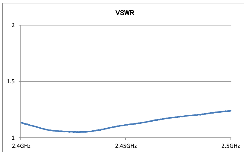
VSWRデータ
