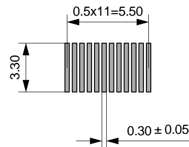
パッド部寸法 (Scale 4:1)
