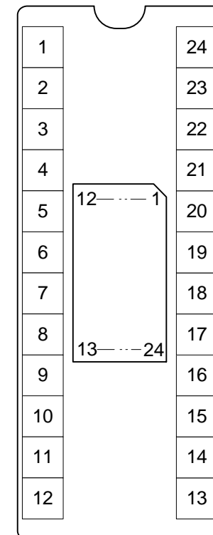
ピン番号図 (Top View) (Out of Scale)
