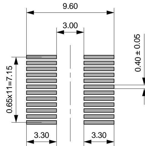
パッド部寸法 (Scale 4:1)
