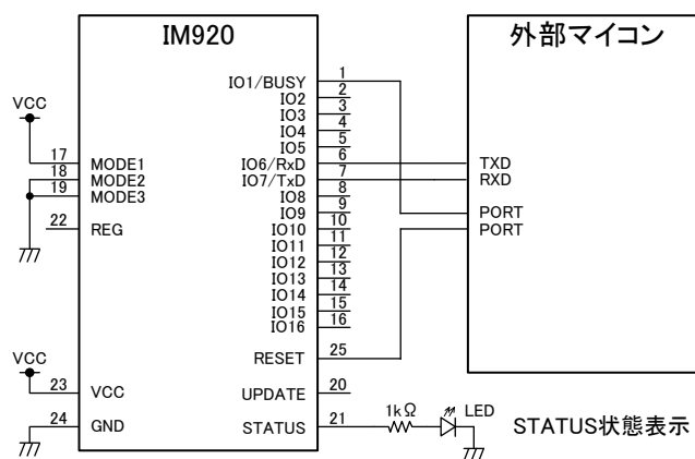
図 10 送受信：データモードの接続例
