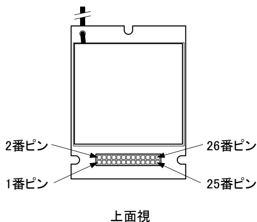
図 1 1 IM920 端子配置図
