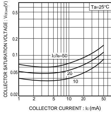
Fig.4 コレクタ・エミッタ飽和電圧 -コレクタ電流特性 (I)
