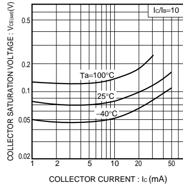
Fig.5 コレクタ・エミッタ飽和電圧 -コレクタ電流特性 (II)
