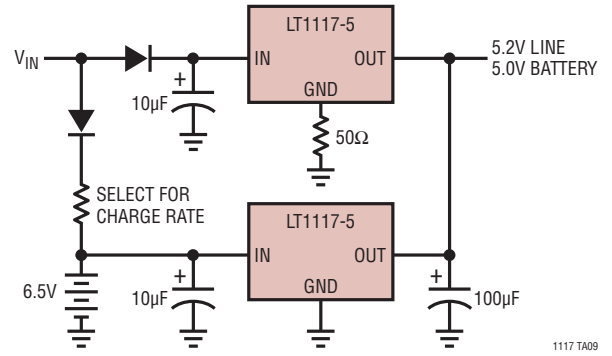
バッテリー・バックアップ付き安定化電源
