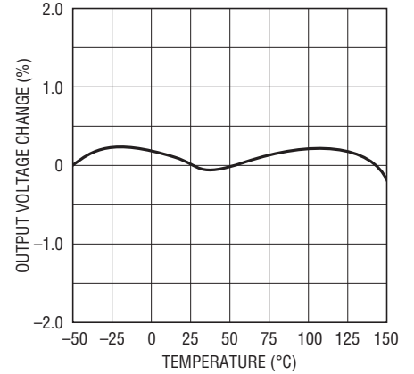
温度安定性
