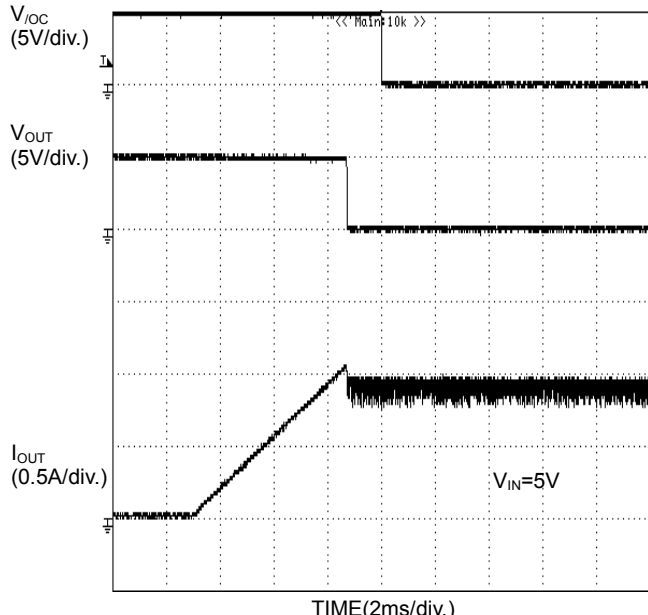
TIME(2ms/div.) Figure 32. 過電流検出特性 ランプ出力 (BD2041AFJ)
