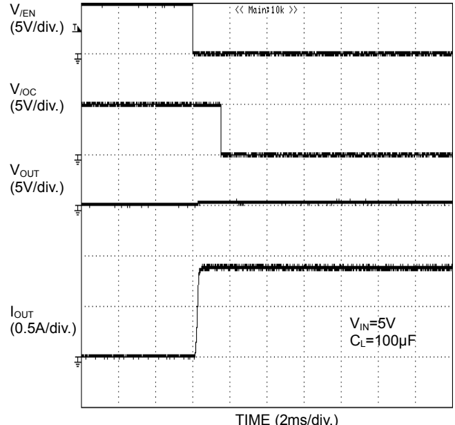
TIME (2ms/div.) Figure 33. 過電流検出特性 ショート状態への Enable (BD2041AFJ)
