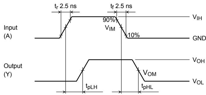
図2 t_{pLH} , t_{pHL}
