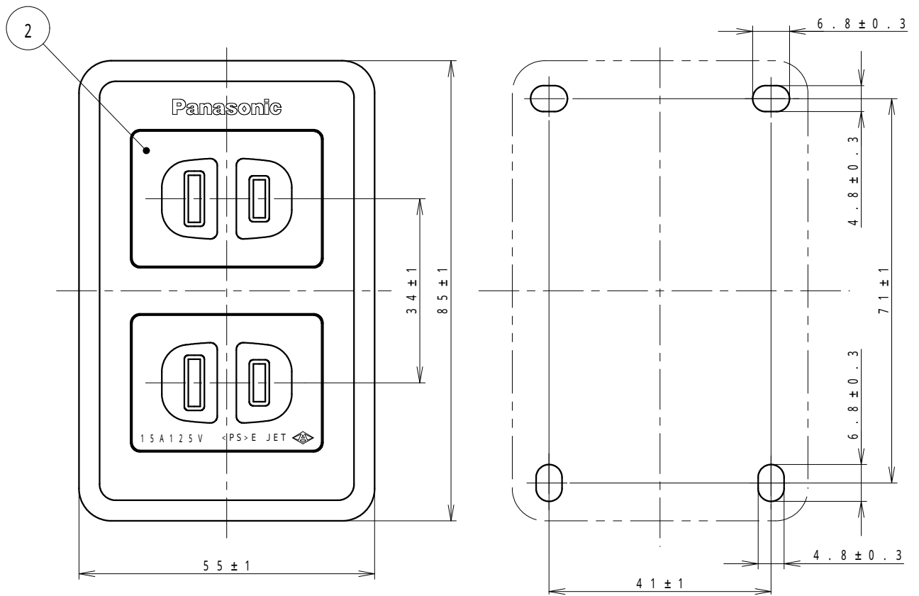
取付寸法
