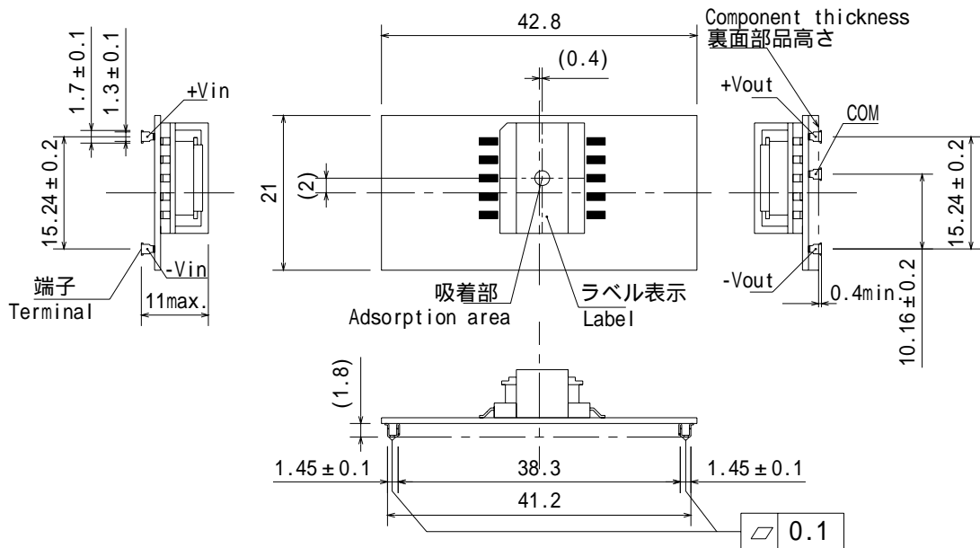
OGD10-**-****-X 推奨加工図 (TOP VIEW)
