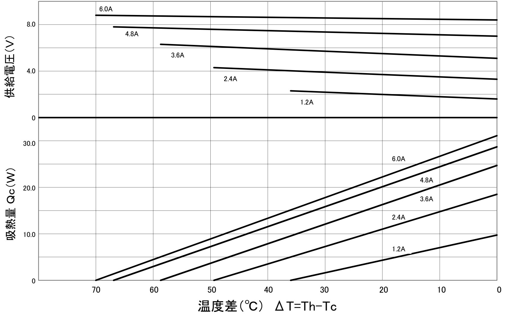
FPH1-7107AC 特性図 (Th=27°C)
