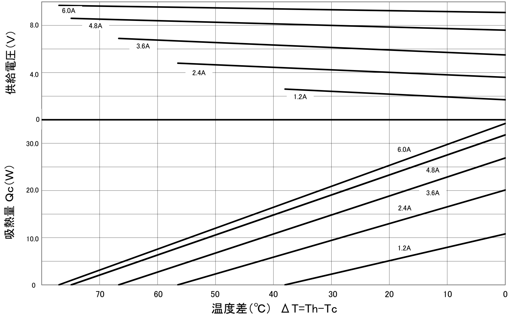
FPH1-7107AC特性図(Th=50°C)
