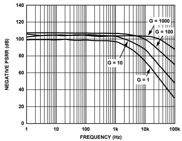
図 26.負の PSRR の周波数特性、 \pm 5 V_S
