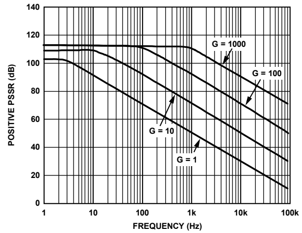
図 24.正の PSRR の周波数特性、 \pm 5 V_S
