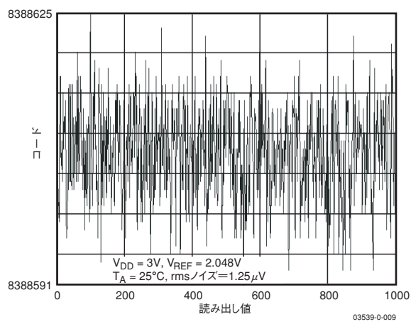
図8. AD7789のノイズ・プロット
