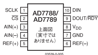
図5. ピン配置
