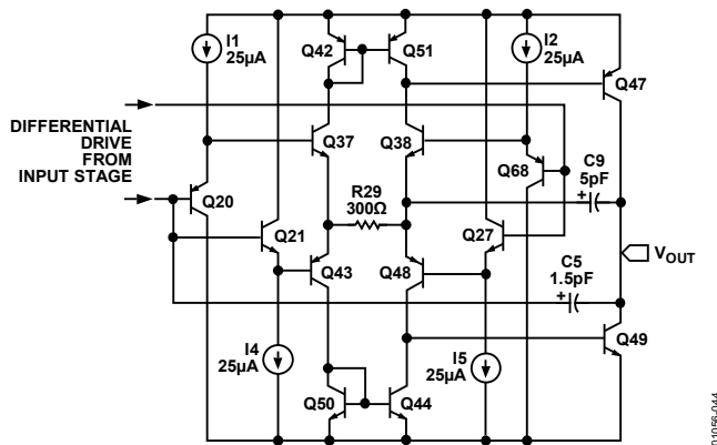
図44. 出力ステージの簡略化した回路図
