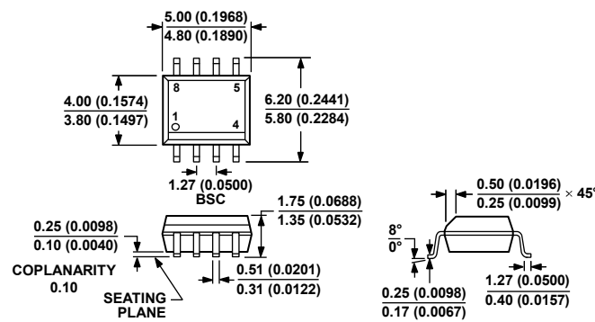
図54.8 ピン・プラスチック・デュアルインライン・パッケージ[PDIP] ナロー・ボディ(N-8) 寸法:インチ(mm)
