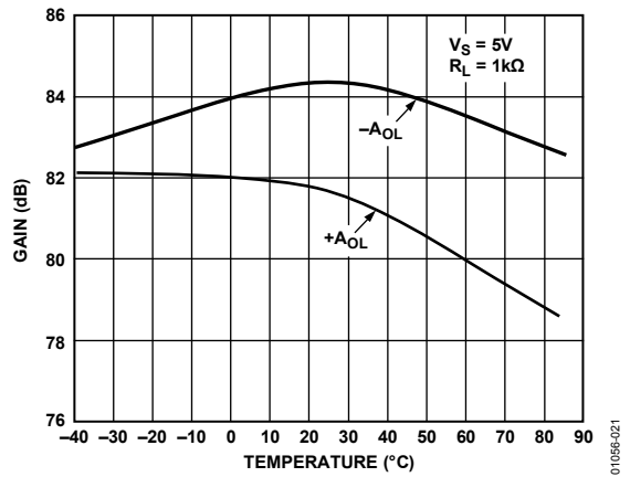
図21. オープン・ループ・ゲイン(A OL )の温度特性
