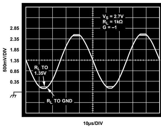
図40.出力振幅
