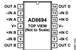
図 5.14 ピン SOIC
