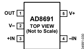
図 1.5 ピン TSOT
