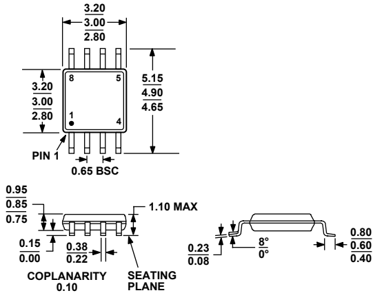
図 34.8 ピン・ミニ・スモール・アウトライン・パッケージ[MSOP] (RM-8) 寸法: mm
