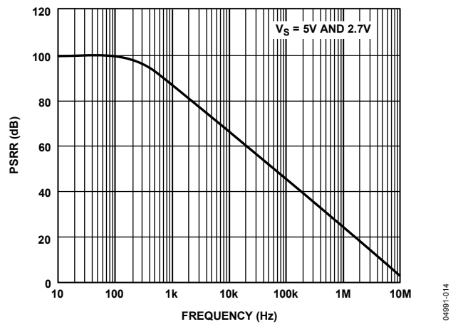
図 18.PSRR の周波数特性
