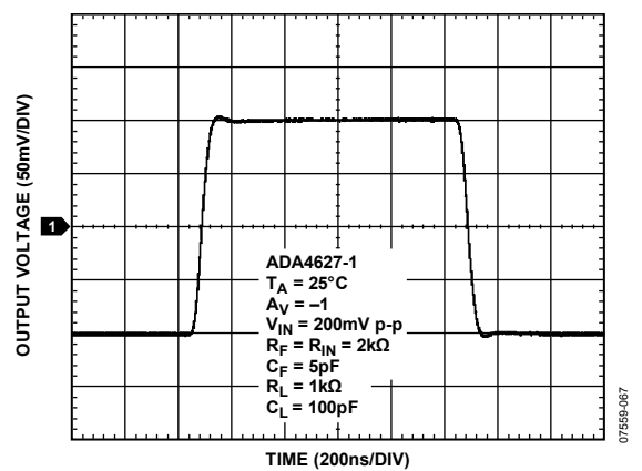
图 33.小信号过渡应答
