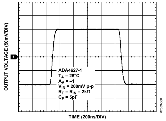
图 31.小信号过渡应答
