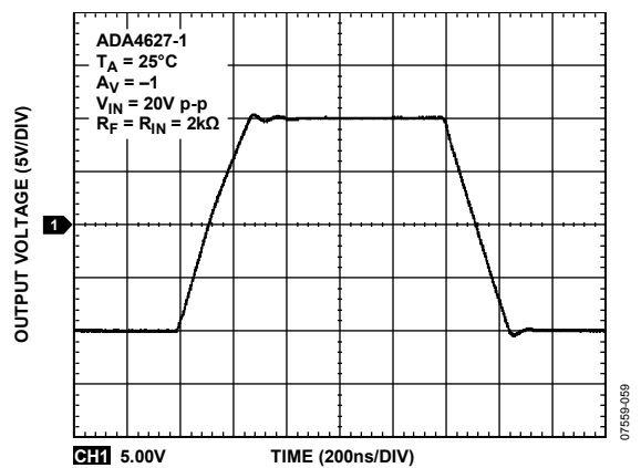
図 27. 大信号過渡応答
