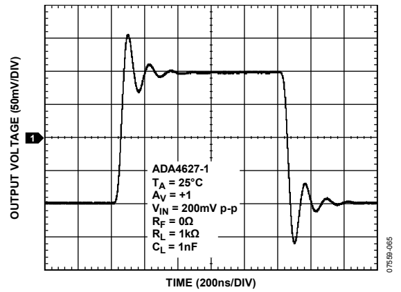
图 32.小信号过渡应答
