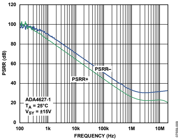
図 10. PSRR の周波数特性
