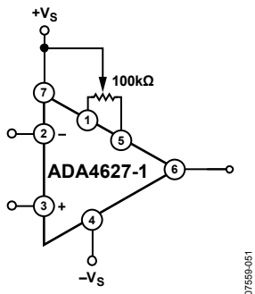
図 46.標準オフセット・ヌル回路
