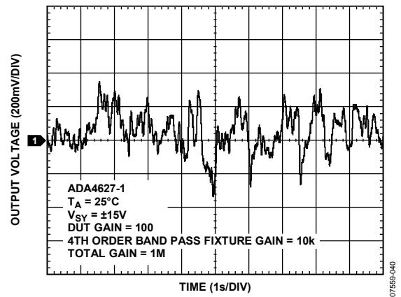
図 38. 0.1~10 Hz でのノイズ
