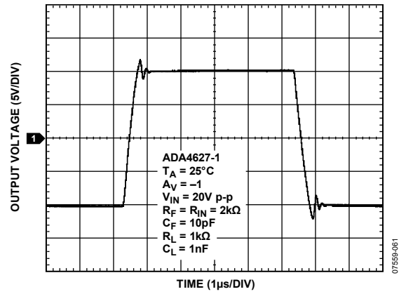
図 25. 大信号過渡応答
