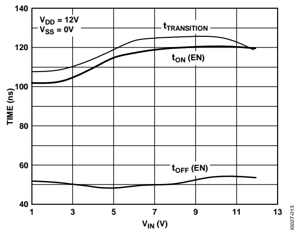
図13.スイッチング時間対 V_{IN} (単電源)
