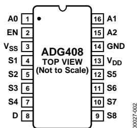
図2.ADG408のピン配置
