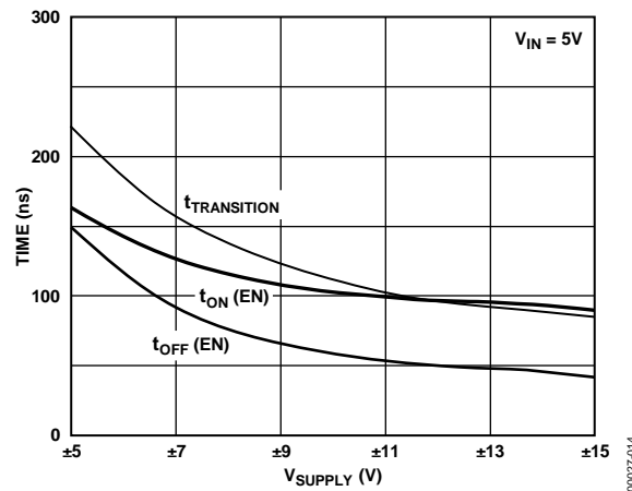
図14.スイッチング時間対両電源電圧
