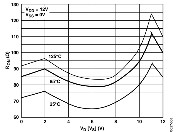
図8. さまざまな温度での、 V_D ( V_S )の関数としての R_{ON}
