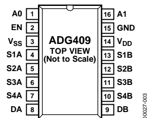
図3.ADG409のピン配置
