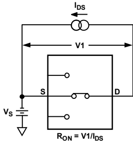
図18. オン抵抗
