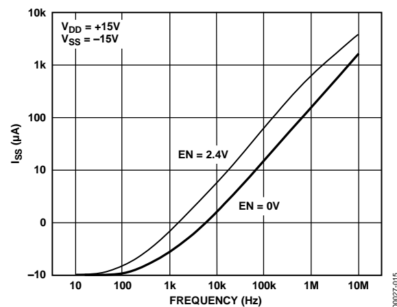
図15.負電源電流対スイッチング周波数
