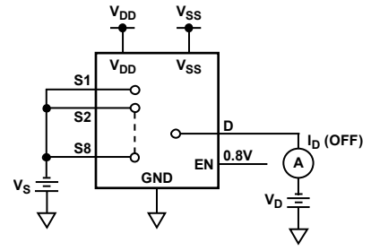
図20. I_D (OFF)
