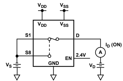
図21. I_D (ON)
