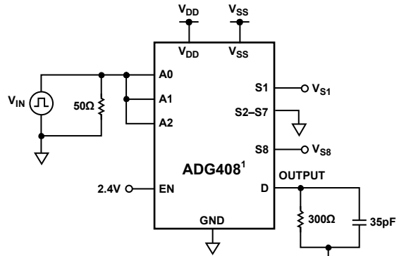
図22. マルチプレクサのスイッチング時間 t_{TRANSITION}
