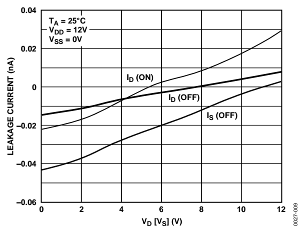
図9. V_D ( V_S )の関数としてのリーク電流
