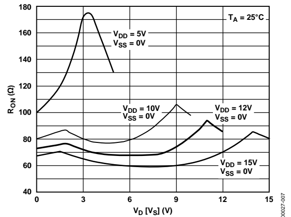
図7. V_D ( V_S )の関数としての R_{ON} :単電源
