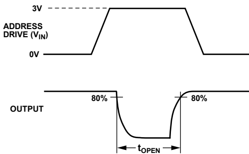
図23. ブレーク・ビフォ・メーカー時間遅延 t_{OPEN}
