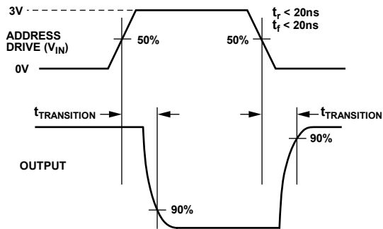
図22. マルチプレクサのスイッチング時間 t_{TRANSITION}
