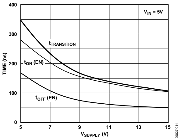
図11.スイッチング時間対単電源電圧
