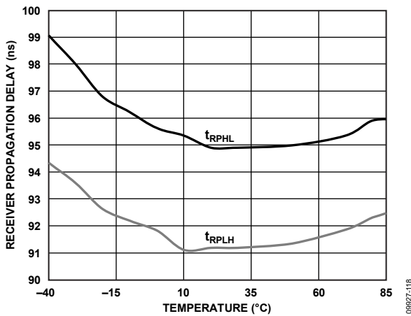
図 22. ADM2687E レシーバ伝搬遅延の温度特性
