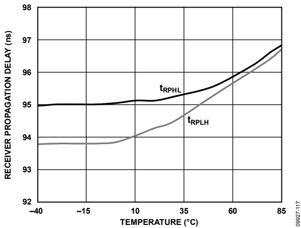
図 21. ADM2682E レシーバ伝搬遅延の温度特性
