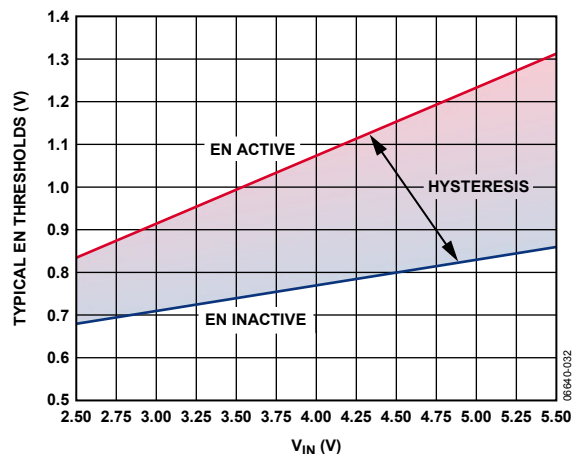
図 32. 入力電圧 対 EN ピンの代表的なスレッショールド値
