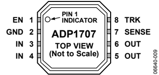
図 7. 8 ピン LFCSP、ADP1707
