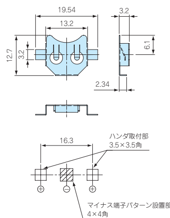
BK-885 外観寸法図
