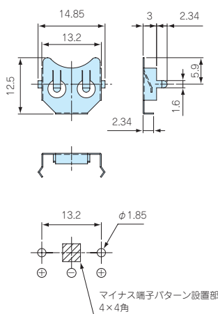
BK-890外観寸法図
