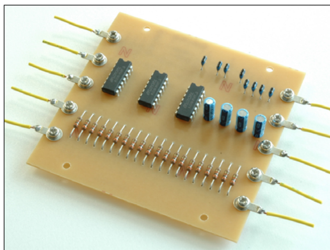
部品実装例
