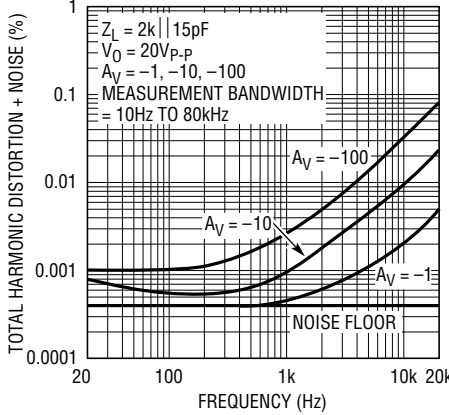
LT1169 • TPC23
