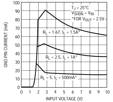
LT1963-2.5 GNDピン電流
