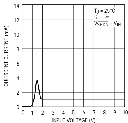
LT1963A-1.8消費電流
