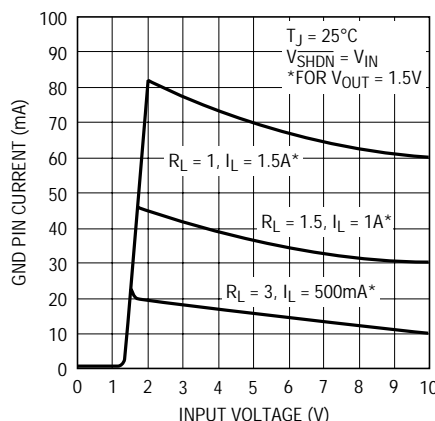
LT1963A-1.5 GNDピン電流
