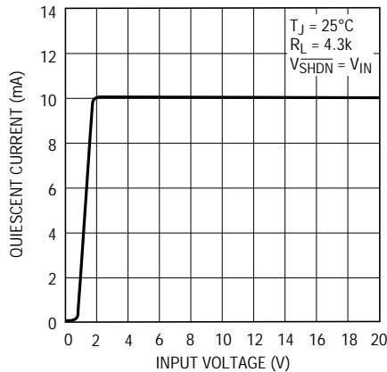
LT1963A消費電流
