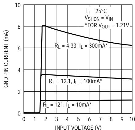
LT1963A GNDピン電流
