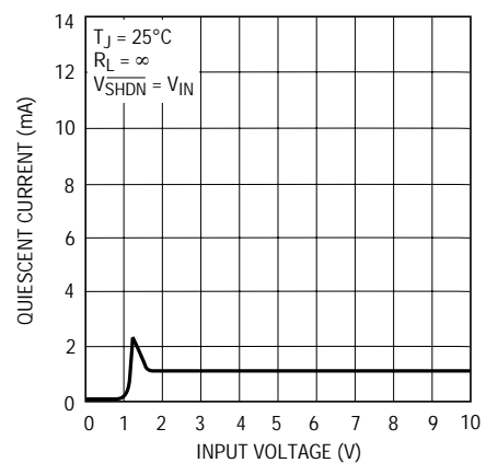
LT1963A-1.5消費電流
