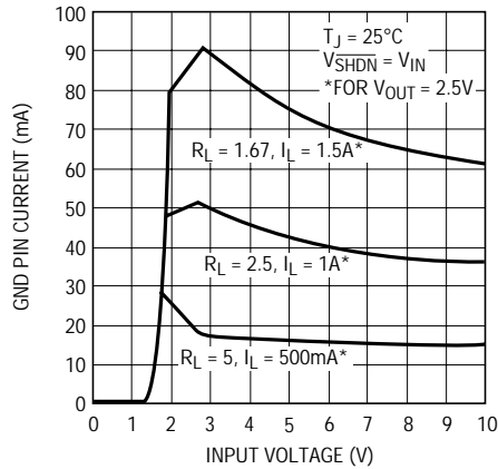
LT1963A-2.5 GNDピン電流
