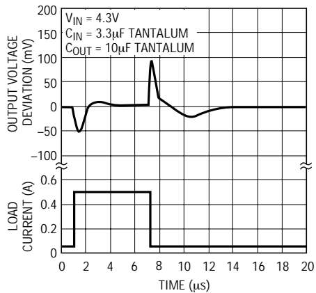
LT1963A-3.3過渡応答
