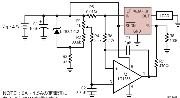
可変電流源
