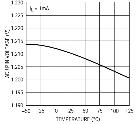
LT1963A ADJピン電圧
