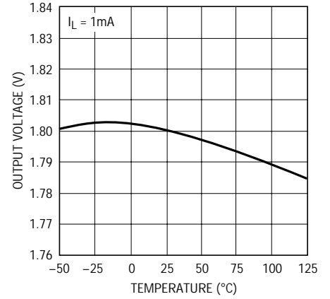
LT1963A-1.8出力電圧
