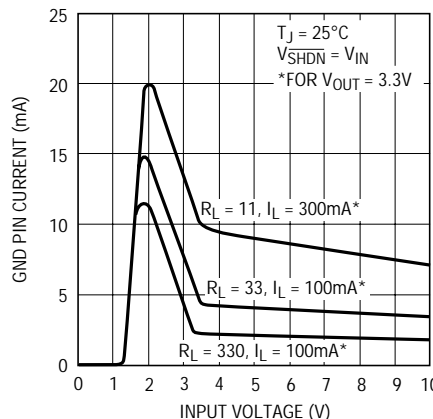
LT1963A-3.3 GNDピン電流
