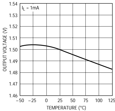
LT1963A-1.5出力電圧
