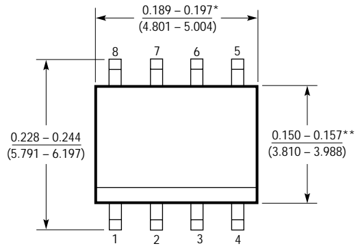
S8パッケージ 8ピン・プラスチックSQ(細型0.150インチ) (Reference LTC DWG # 05-08-1610)
