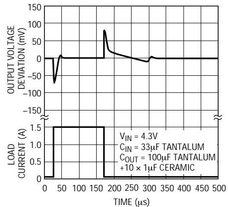
LT1963A-3.3過渡応答
