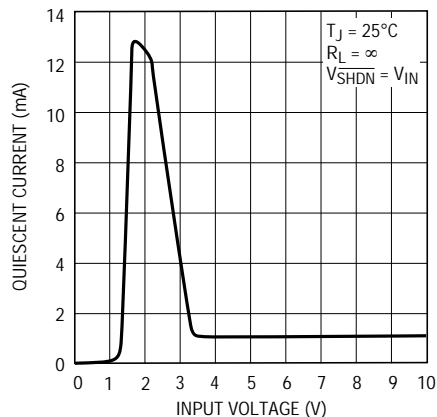
LT1963A-3.3消費電流
