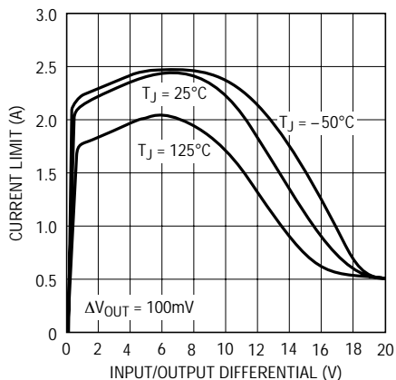
電流制限
