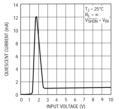
LT1963A-2.5消費電流
