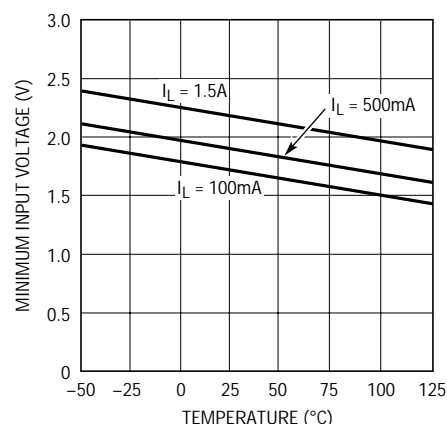
LT1963Aの最小入力電圧
