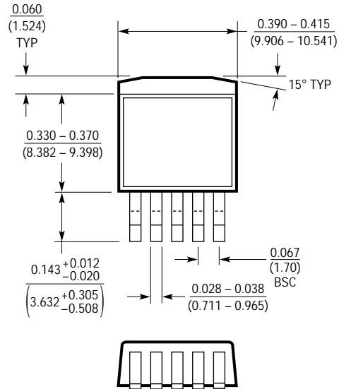
Qパッケージ 5ピン・プラスチックDD Pak (Reference LTC DWG # 05-08-1461)
