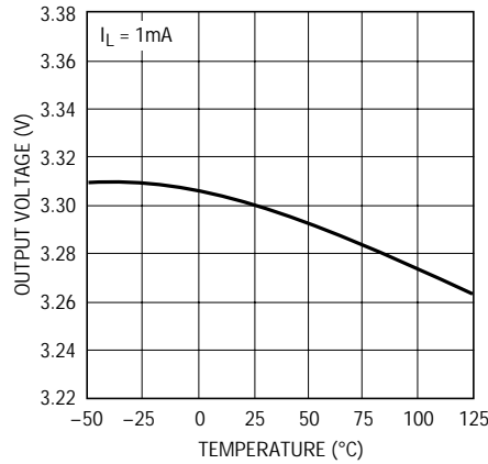
LT1963A-3.3出力電圧
