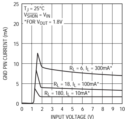
LT1963A-1.8 GNDピン電流
