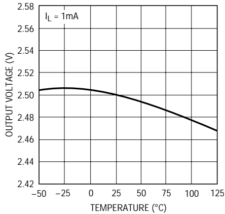
LT1963A-2.5出力電圧
