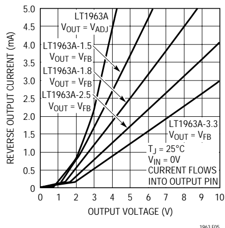
図5. 逆出力電流
