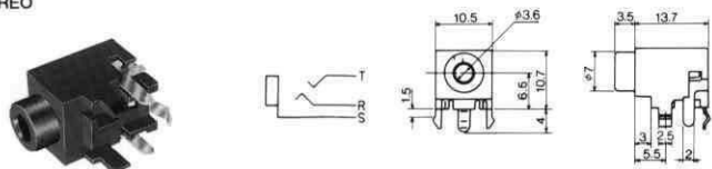
No.MX-362GL (φ3.5) STEREO
