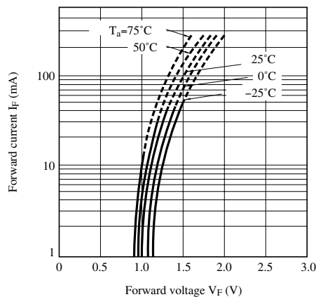
Fig.4 順電流 順電圧特性
