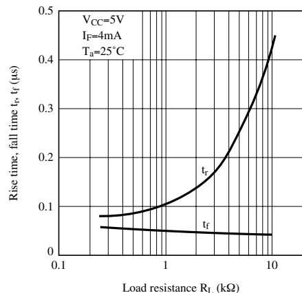
Fig.11 上昇時間・下降時間 負荷抵抗特性
