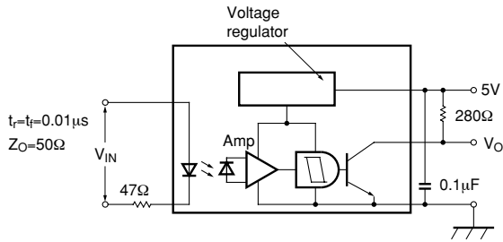
Fig.1 応答時間の測定回路
