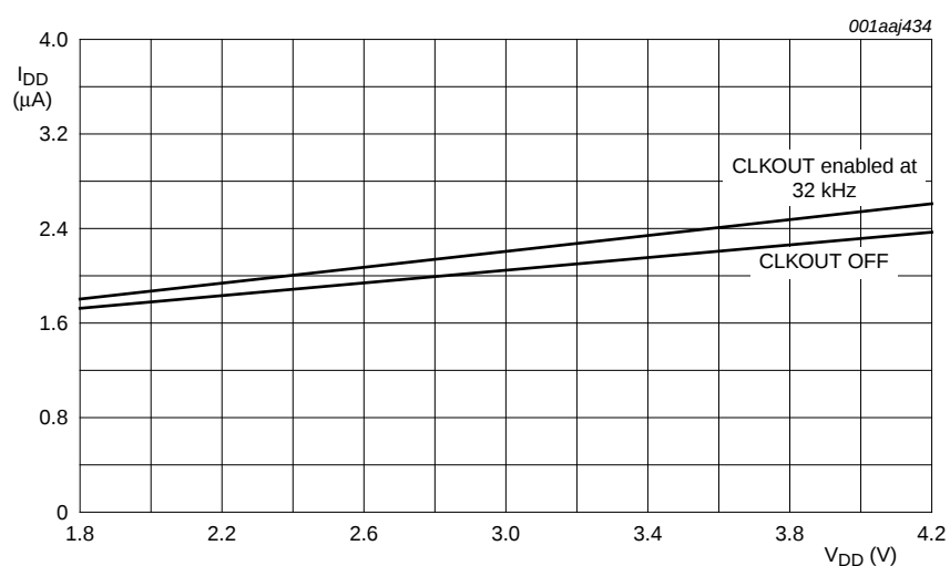
b. PWRMNG[2:0] = 000; TSOFF = 0; T amb = 25 °C; \overline{\text{TS}} input floating
