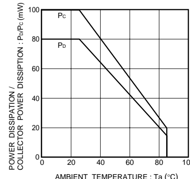
Fig.5 許容・コレクタ損失 - 周囲温度特性
