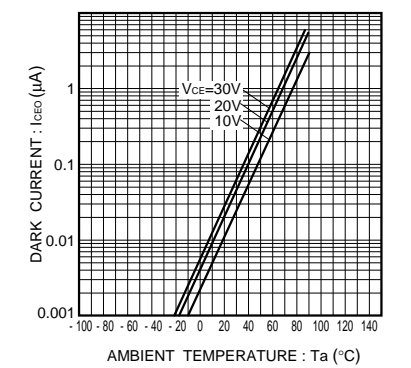
Fig.9 暗電流 - 周囲温度特性
