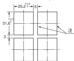
取付穴加工寸法
