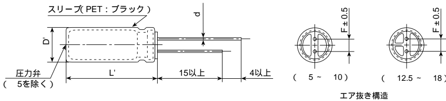
エア抜き構造
