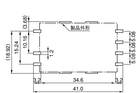
推奨基板取付け寸法
