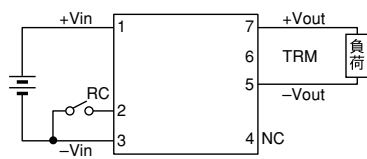
接続図
