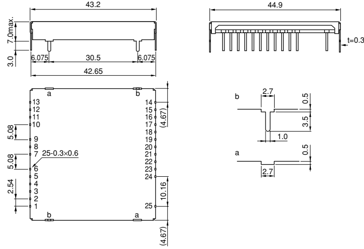
形状・寸法
