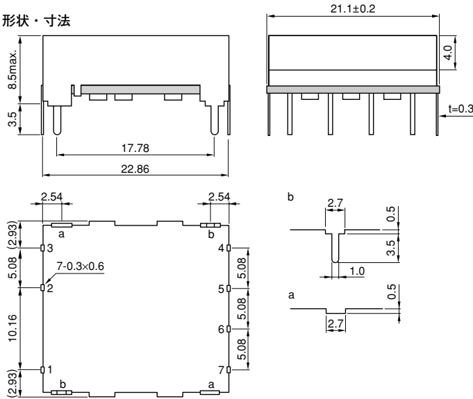
形状・寸法
