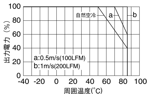
周周温度-出力電力ディレーティング (共通仕様)
