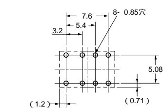
プリント基板加工寸法 (BOTTOM VIEW) 寸法公差は±0.1mmです。
