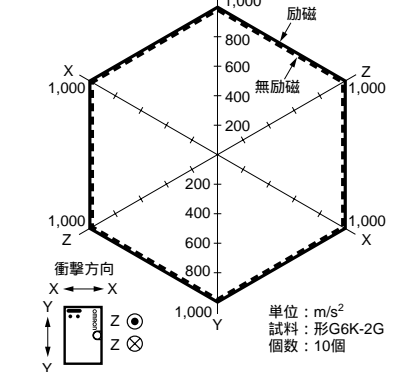
誤動作衝撃
