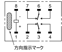
端子配置/内部接続図 (TOP VIEW)
