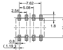
プリント基板加工寸法 (TOP VIEW) 寸法公差は±0.1mmです。
