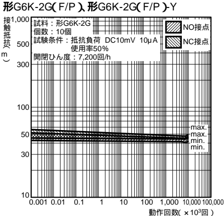
接触信頼性試験 *1, *2
