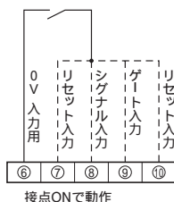
接点ONで動作
