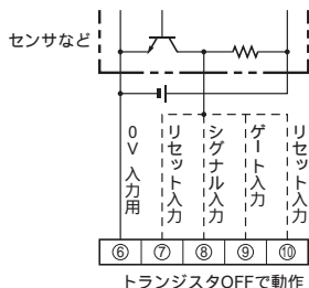
トランジスタOFFで動作
