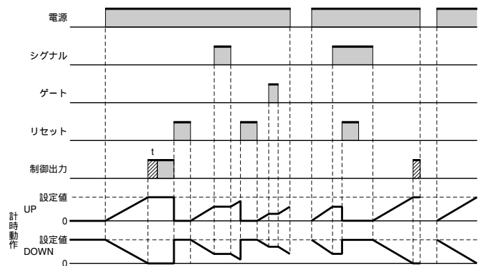
A-3モード(パワーオンディレイ( )): 電源保持動作)
