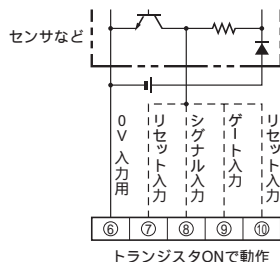
トランジスタONで動作
