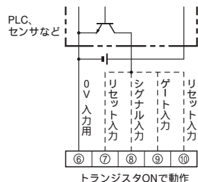
トランジスタONで動作
