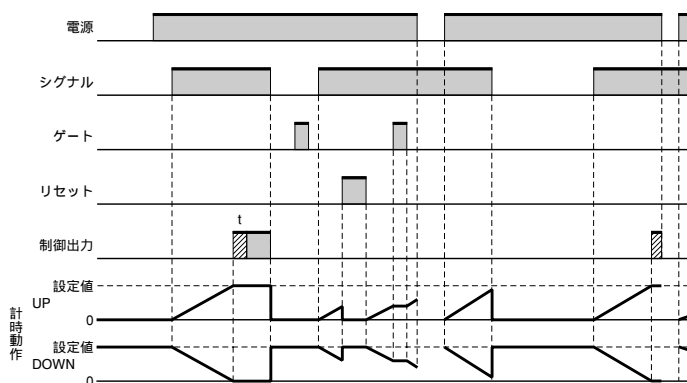
A-2モード(パワーオンディレイ( )): 電源リセット動作)
