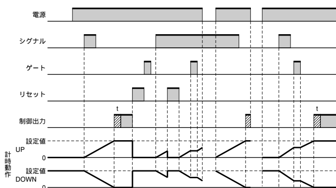
A-1モード(シグナルオンディレイ( )): 電源リセット動作)
