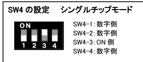
図 3-1 SW4 ジャンパ設定図1
