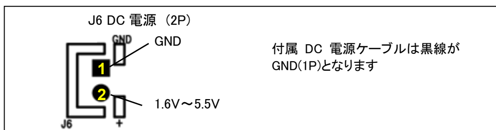
図 2-2 DC 電源図
