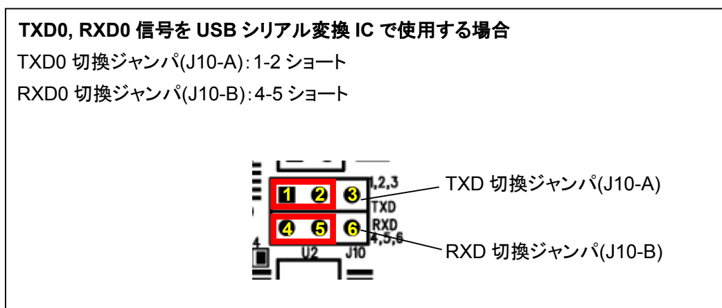
図 2-3 J10-A, J10-B ジャンパ設定例
