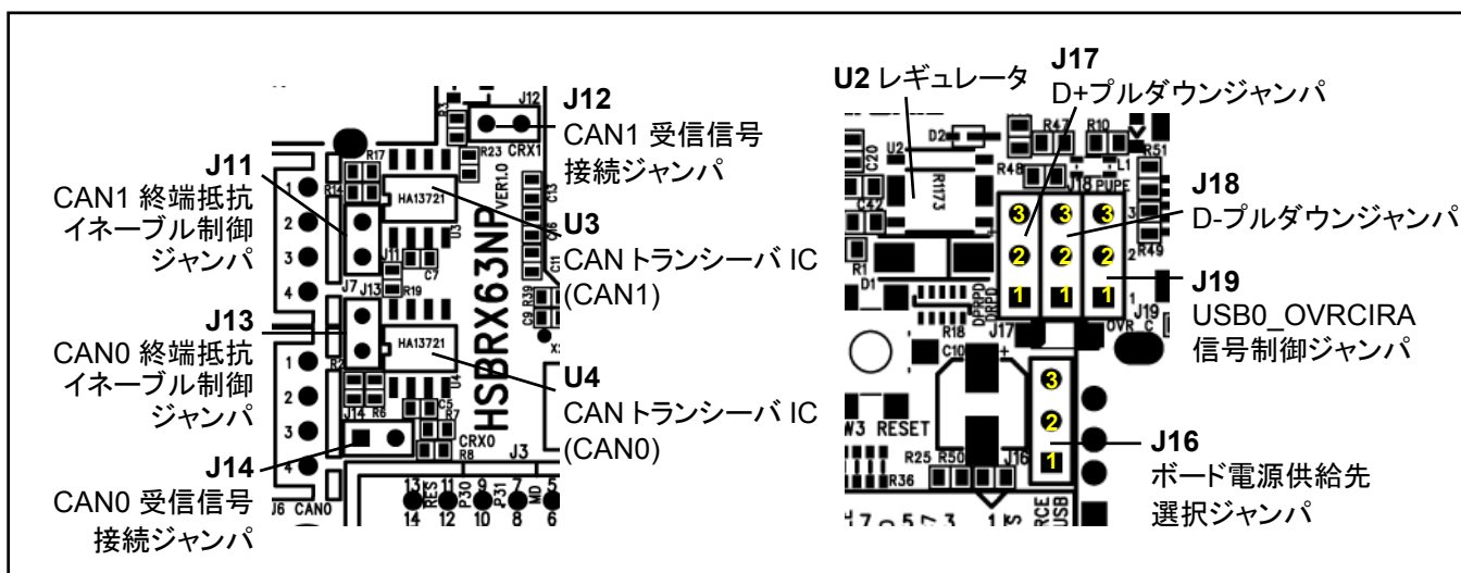
図 1-2 ボード配置図(補足図)
