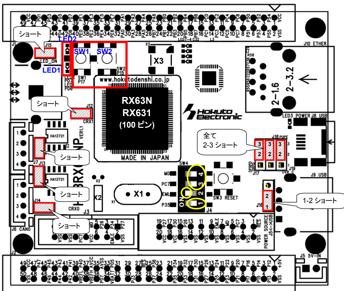
図 5-1 初期設定図
