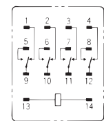
端子配置/内部接続図 (BOTTOM VIEW)
