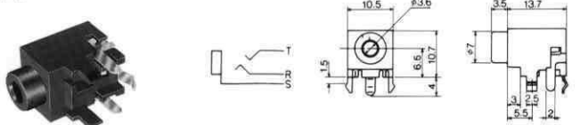
No.MX-362GL (φ3.5) STEREO
