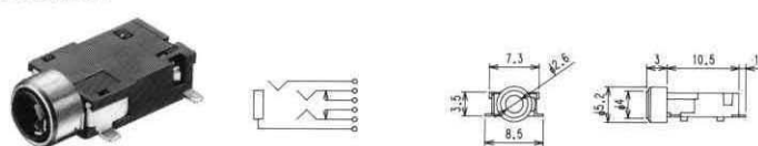
No.M02-787A (φ2.5) 4-CONDUCTOR
