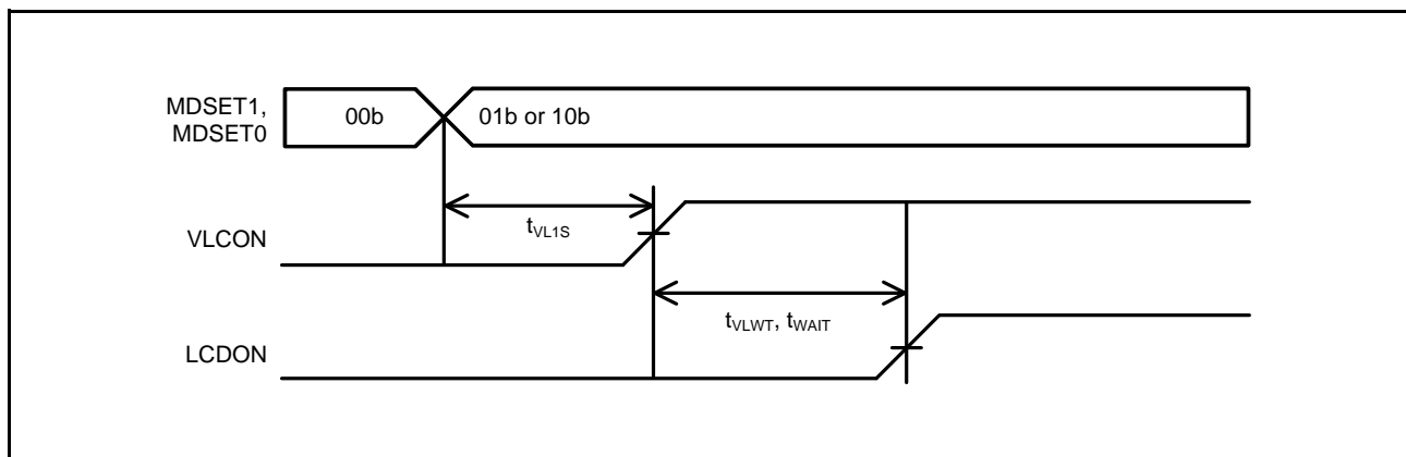
図 5.61 LCD 基準電圧セットアップ時間と昇圧ウェイト時間と容量分割ウェイト時間
