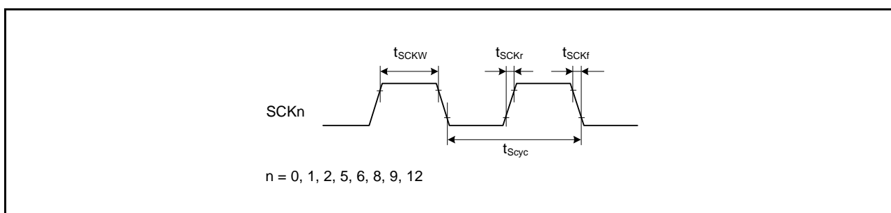
図 5.38 SCK クロック入力タイミング
