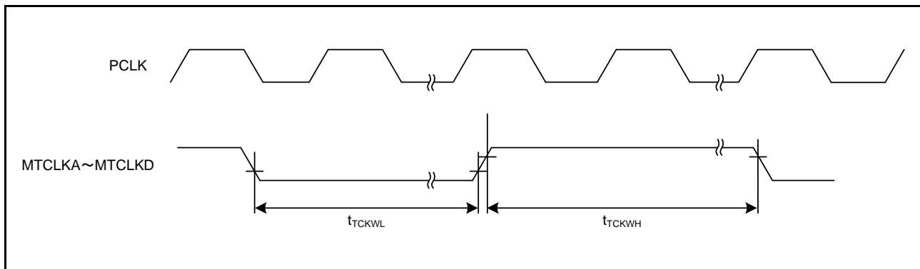
図 5.35 MTU2 クロック入力タイミング
