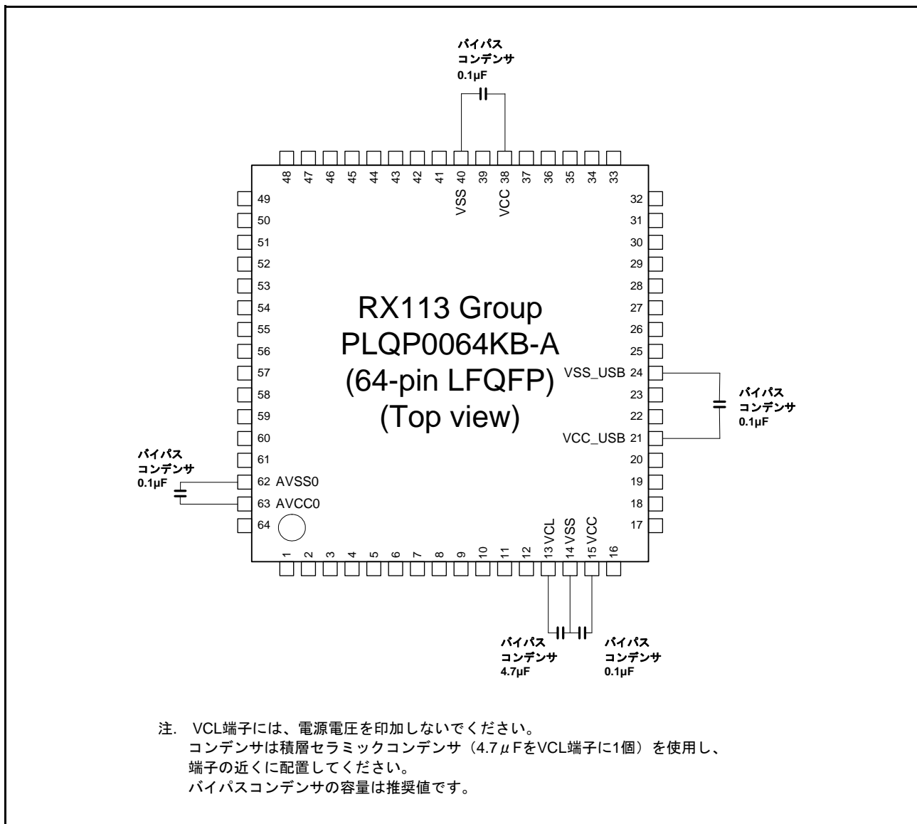
図 5.68 コンデンサ接続方法（64ピン）
