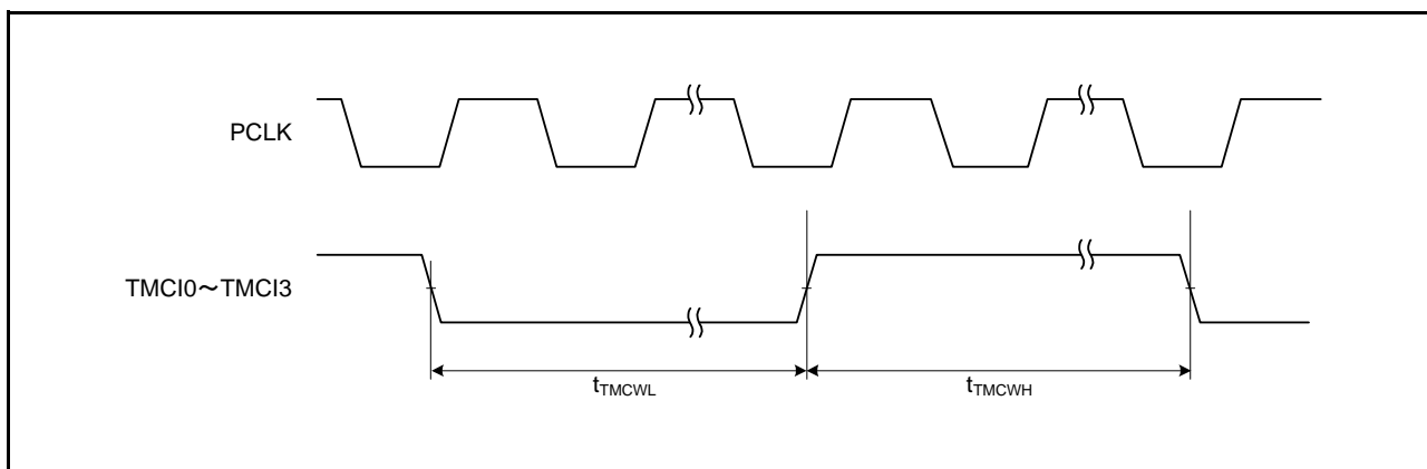
図 5.37 TMR クロック入力タイミング
