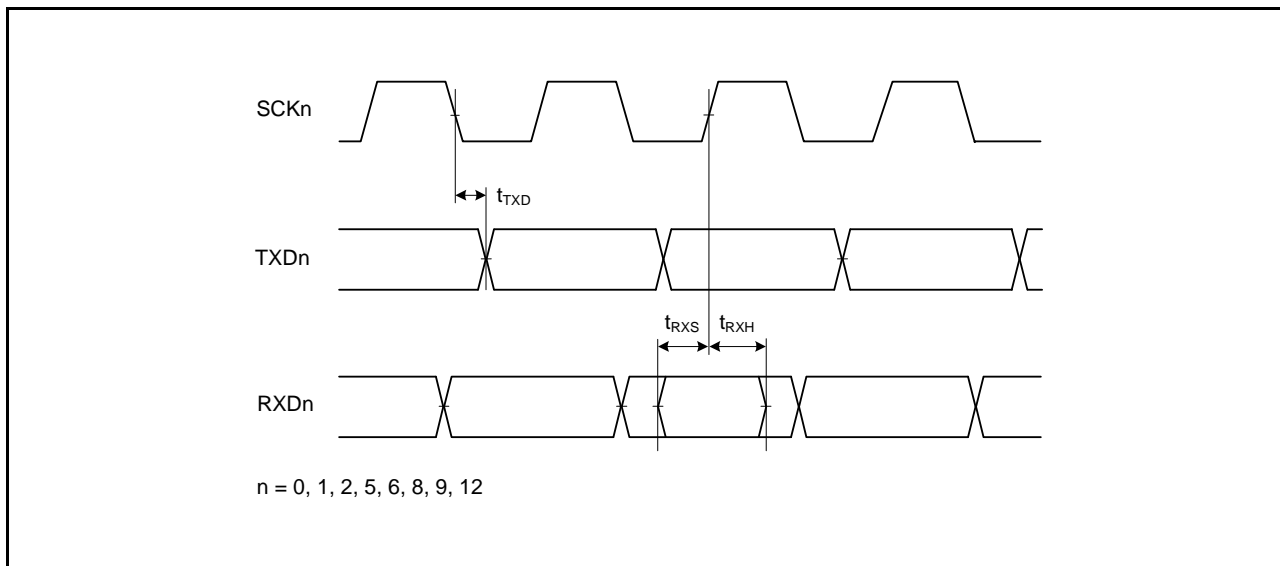
図 5.39 SCI 入出力タイミング / クロック同期式モード
