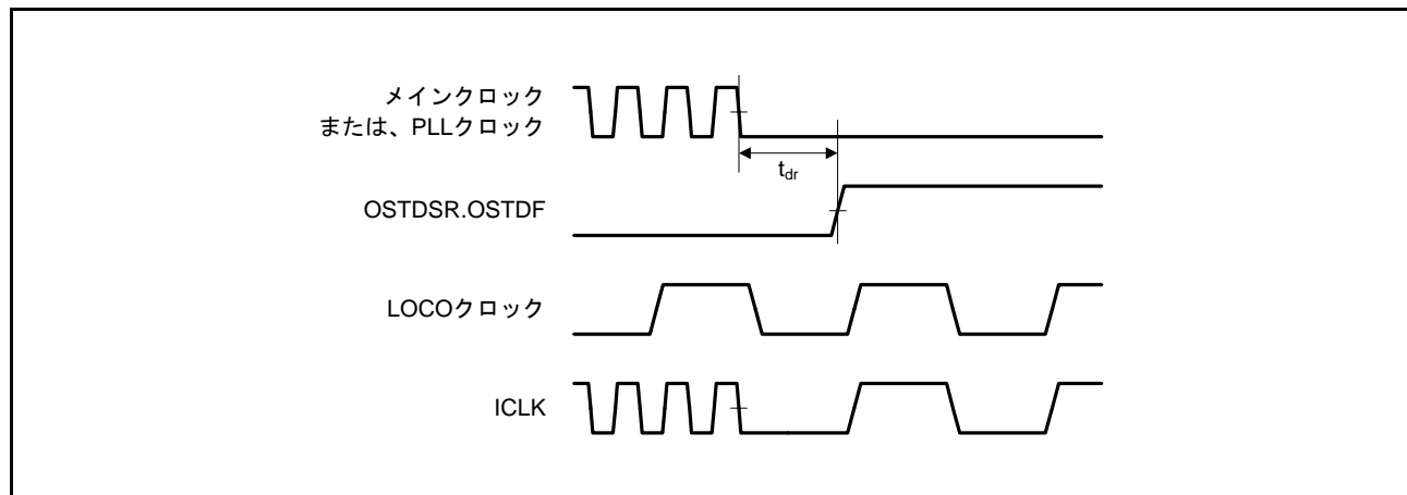
図 5.66 発振停止検出タイミング
