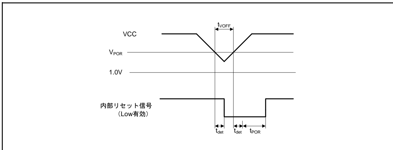
図 5.62 電圧検出リセットタイミング
