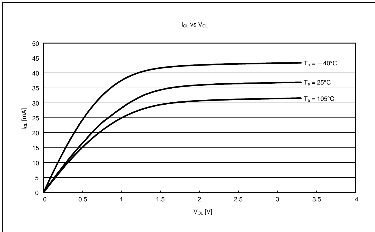
図 5.13 RIIC 出力端子の V_{OL} 、 I_{OL} 温度特性 V_{CC} = 3.3\text{V} (参考データ)
