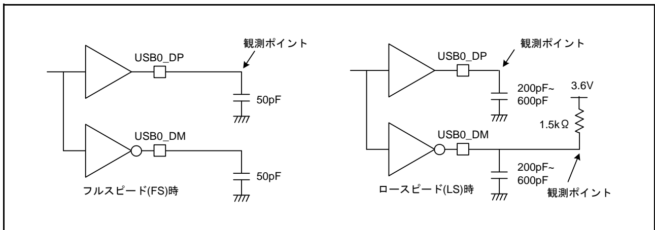
図 5.55 測定回路
