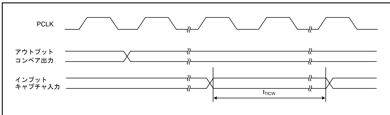
図 5.34 MTU2 入出力タイミング
