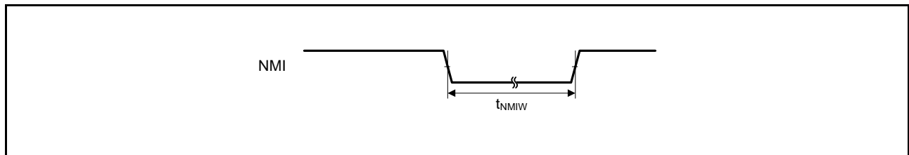
図 5.31 NMI 割り込み入カタイミング
