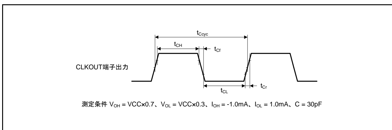
図 5.41 CLKOUT 出カタイミング
