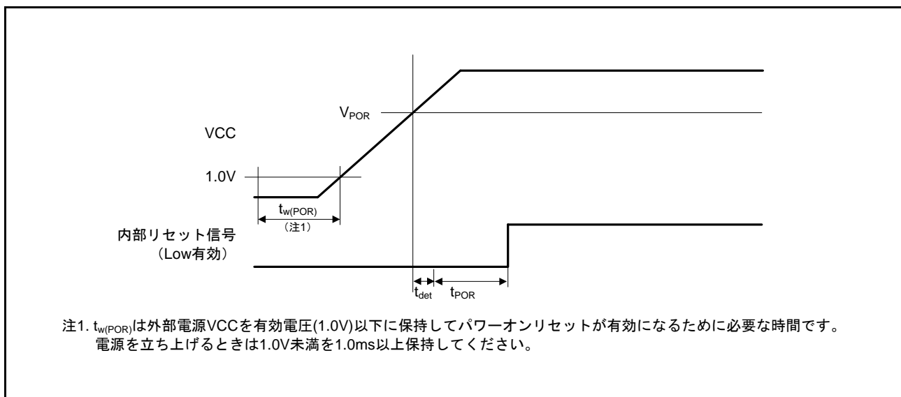
図 5.63 パワーオンリセットタイミング
