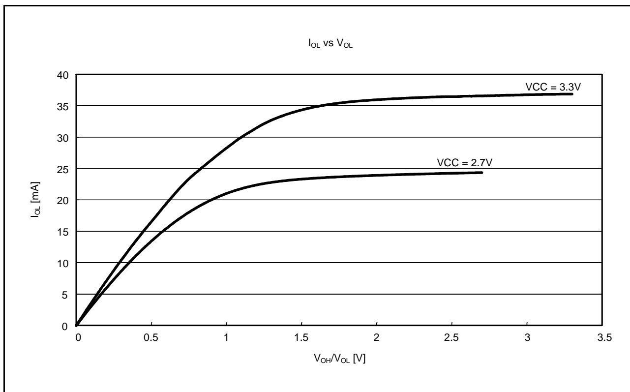
図 5.11 RIIC 出力端子の V OL 、I OL 電圧特性 T a = 25 °C (参考データ)
