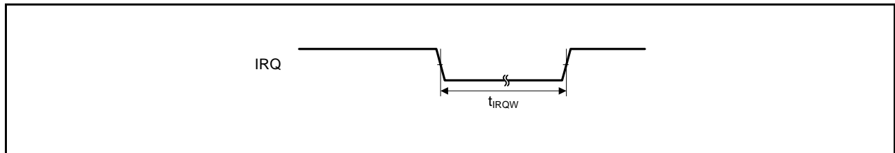
図 5.32 IRQ 割り込み入カタイミング
