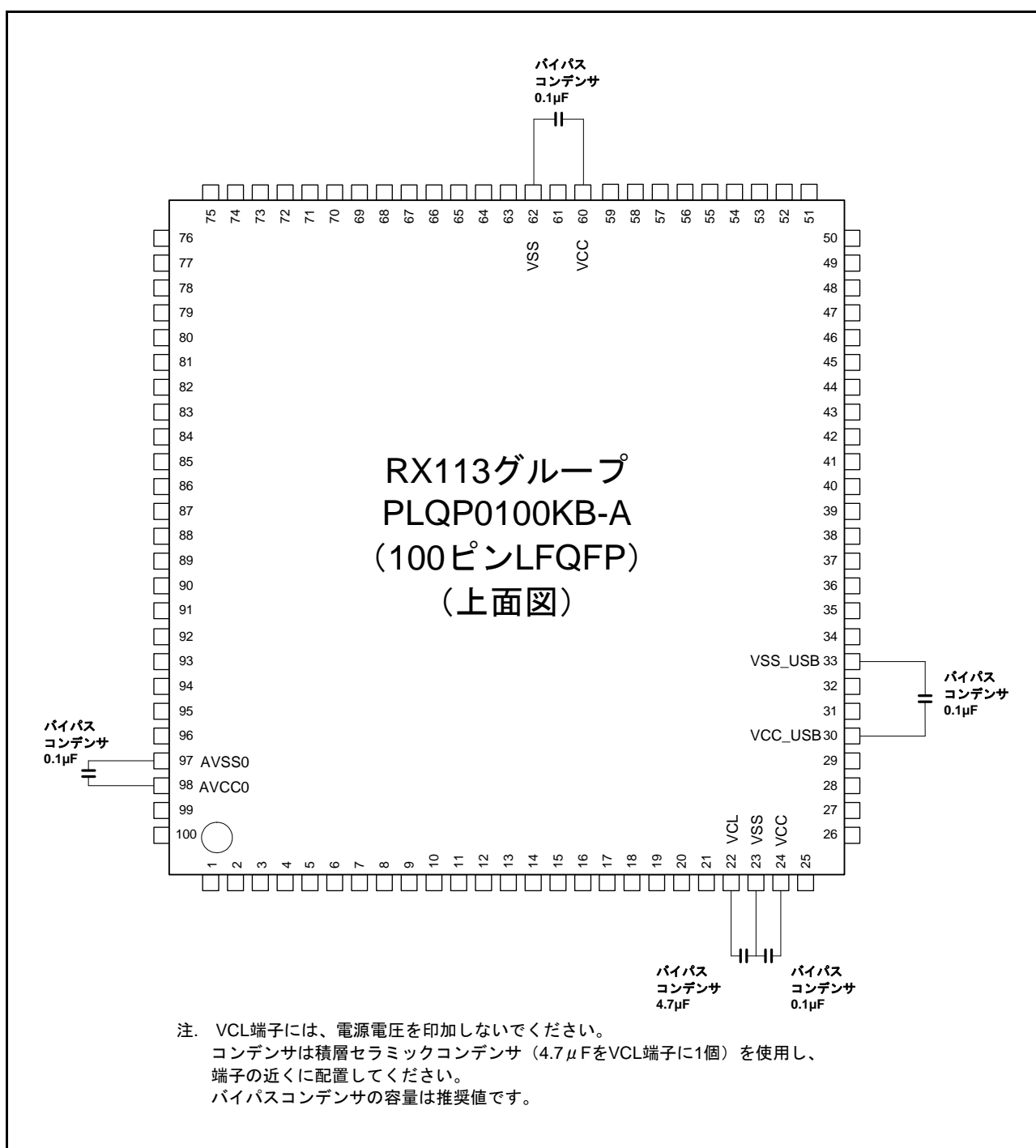
図 5.67 コンデンサ接続方法（100ピンLFQFP）
