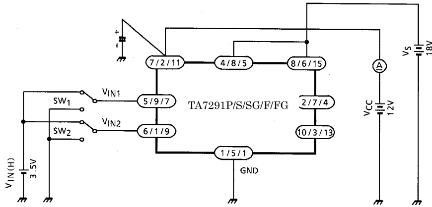
TA7291F/FG の FIN は GND ショート
