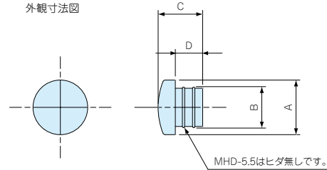
外観寸法図
