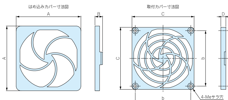
HF-P80・HF-P90・HF-P120 ※図面はHF-P80
