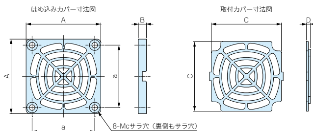
HF-P80・HF-P90・HF-P120 ※図面はHF-P80
