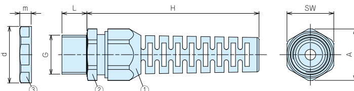
外観寸法図
