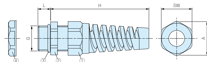
外観寸法図
