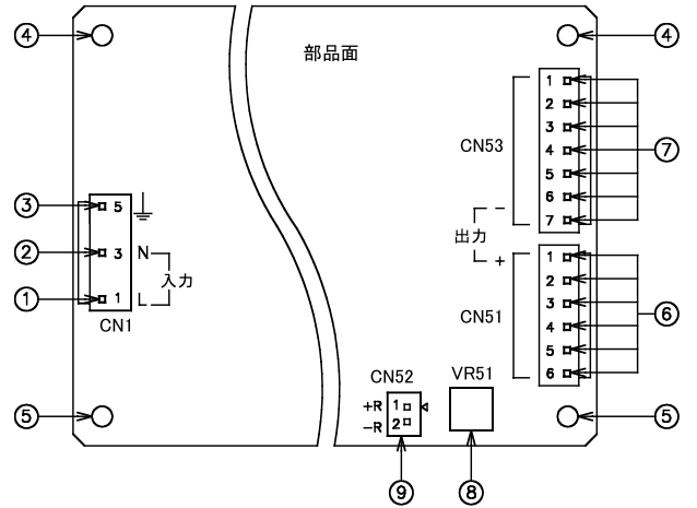
ZWS150BAF
