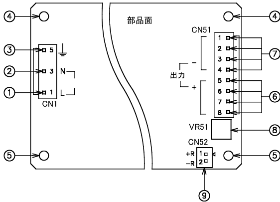
ZWS300BAF
