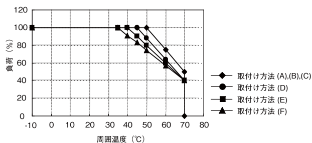
ZWS50BAF
