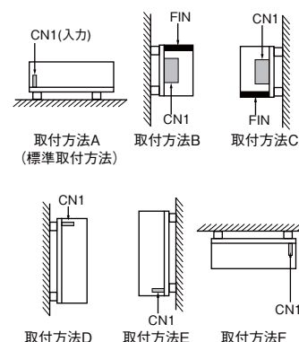
【標準仕様、/CO2、/FV、/A、/L (強制空冷)】
