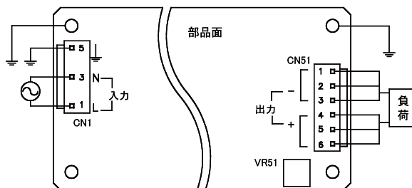
ZWS75BAF
