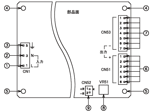
ZWS150BAF
