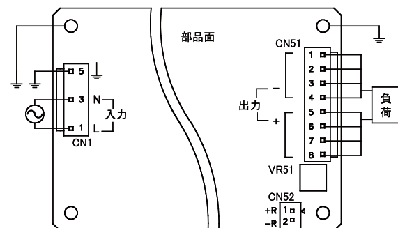
ZWS100BAF
