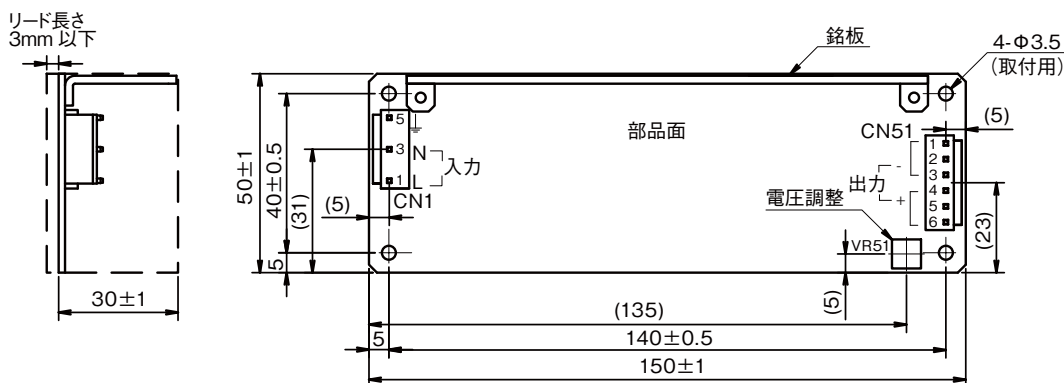
[ZWS75BAF標準仕様、/CO2、/FV]
