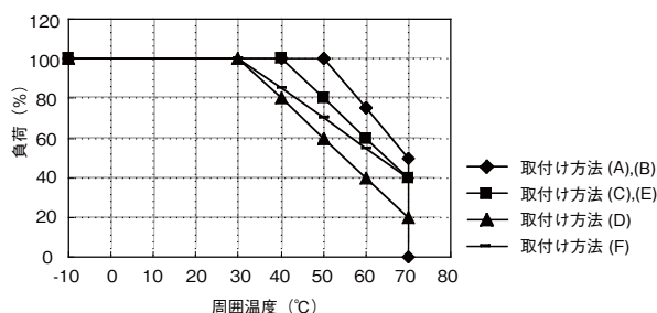
ZWS100BAF、ZWS150BAF
