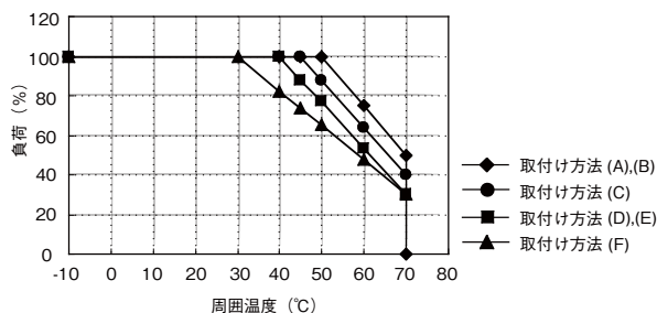
ZWS75BAF
