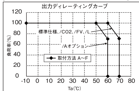
[標準仕様、/CO2、/FV、/A、/L (強制空冷)]
