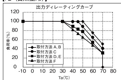
【/L (自然空冷)】
