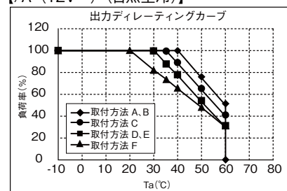
【/A (12V~) (自然空冷)】
