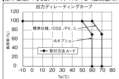
【標準仕様、/CO2、/FV、/A、/L (強制空冷)】
