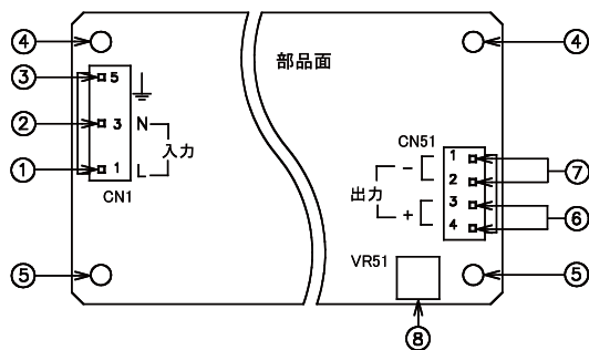
ZWS100BAF
