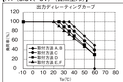
【/A (3.3V、5V) (自然空冷)】
