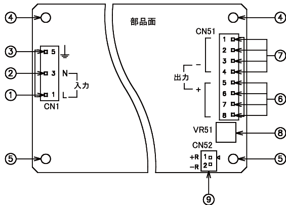
ZWS100BAF
