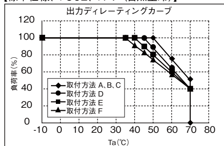
[/L (自然空冷)]
