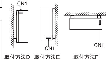
[標準仕様、/CO2、/FV、/A、/L (強制空冷)]
