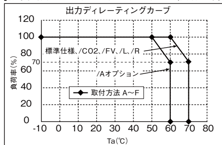
[標準仕様、/CO2、/FV、/A、/L、/R (強制空冷)]
